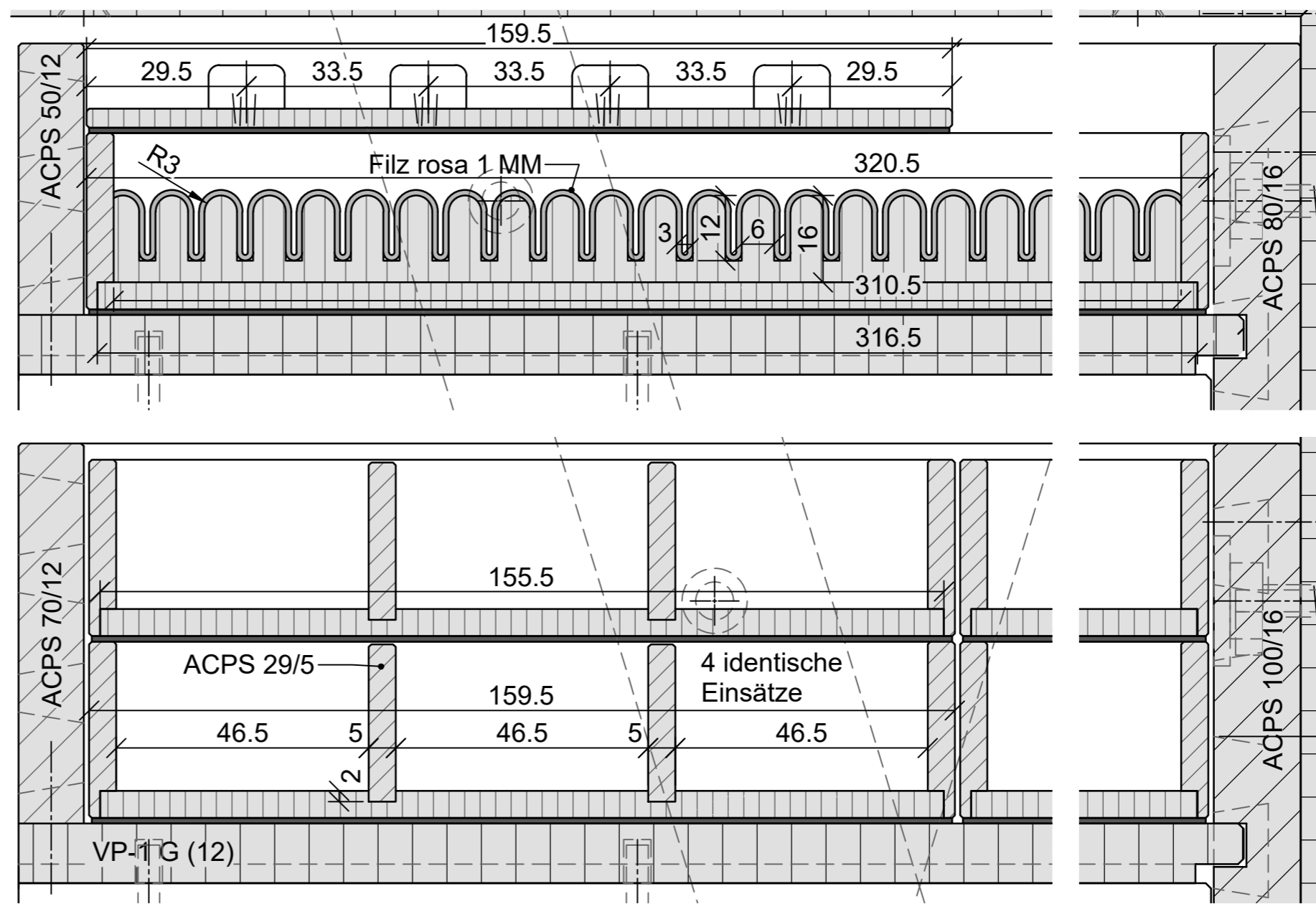
Schnitt B1 M 1:1
