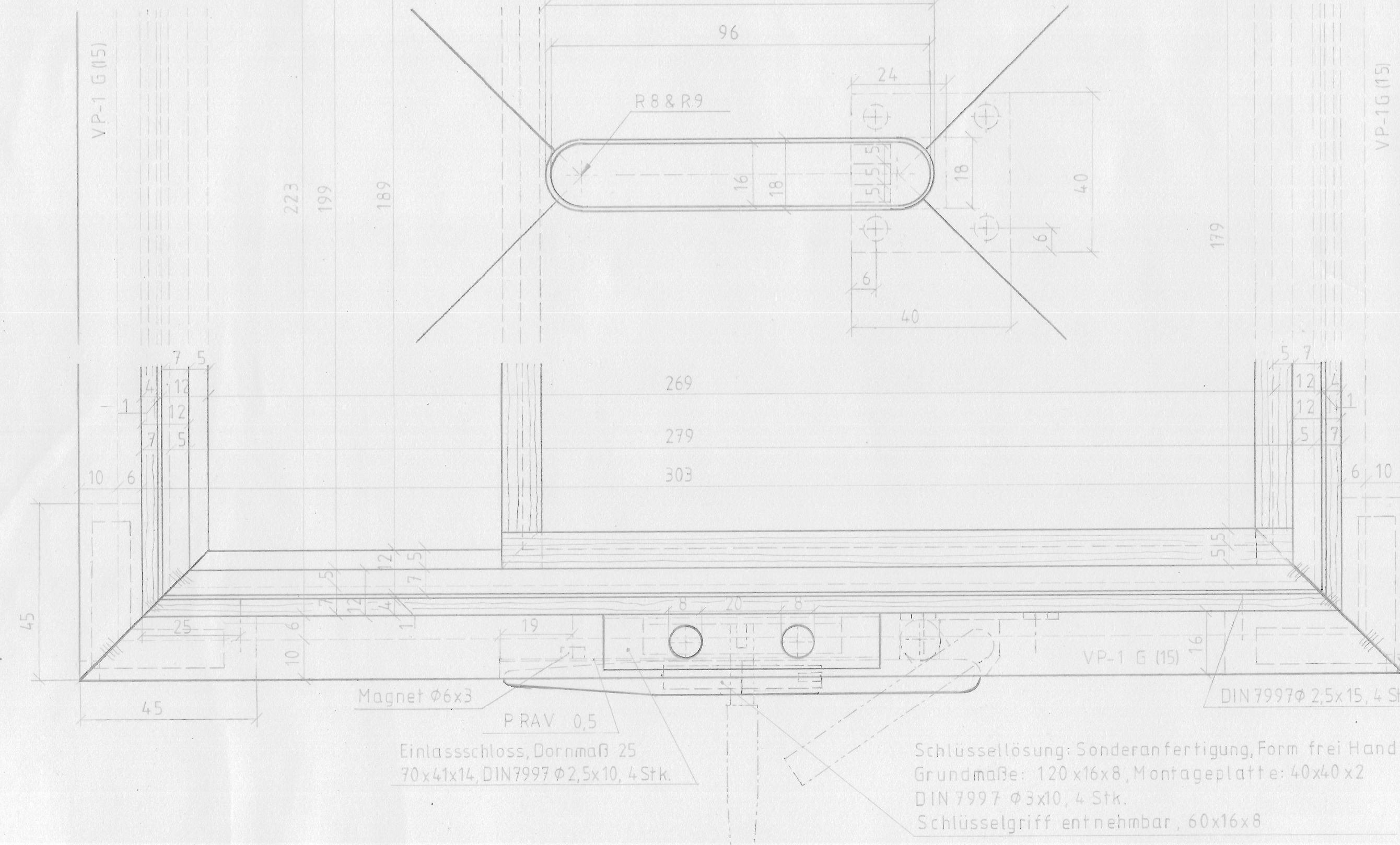
Schnitt A-A
